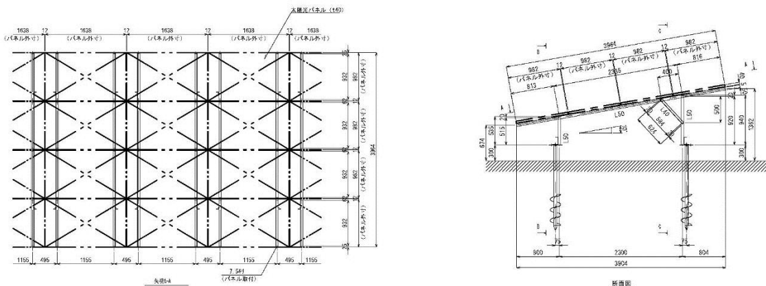
太陽光パネル設置断面図
